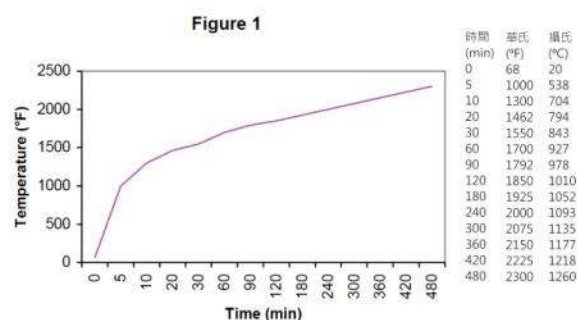
▲ ASTM E152火焰測試溫度曲線圖
